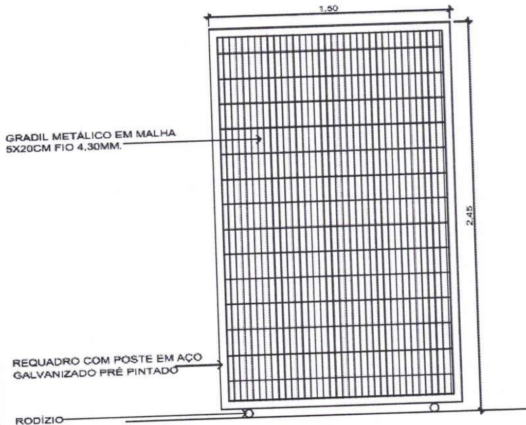
2 DETALHE PORTÃO 09 ESCALA 1/25
